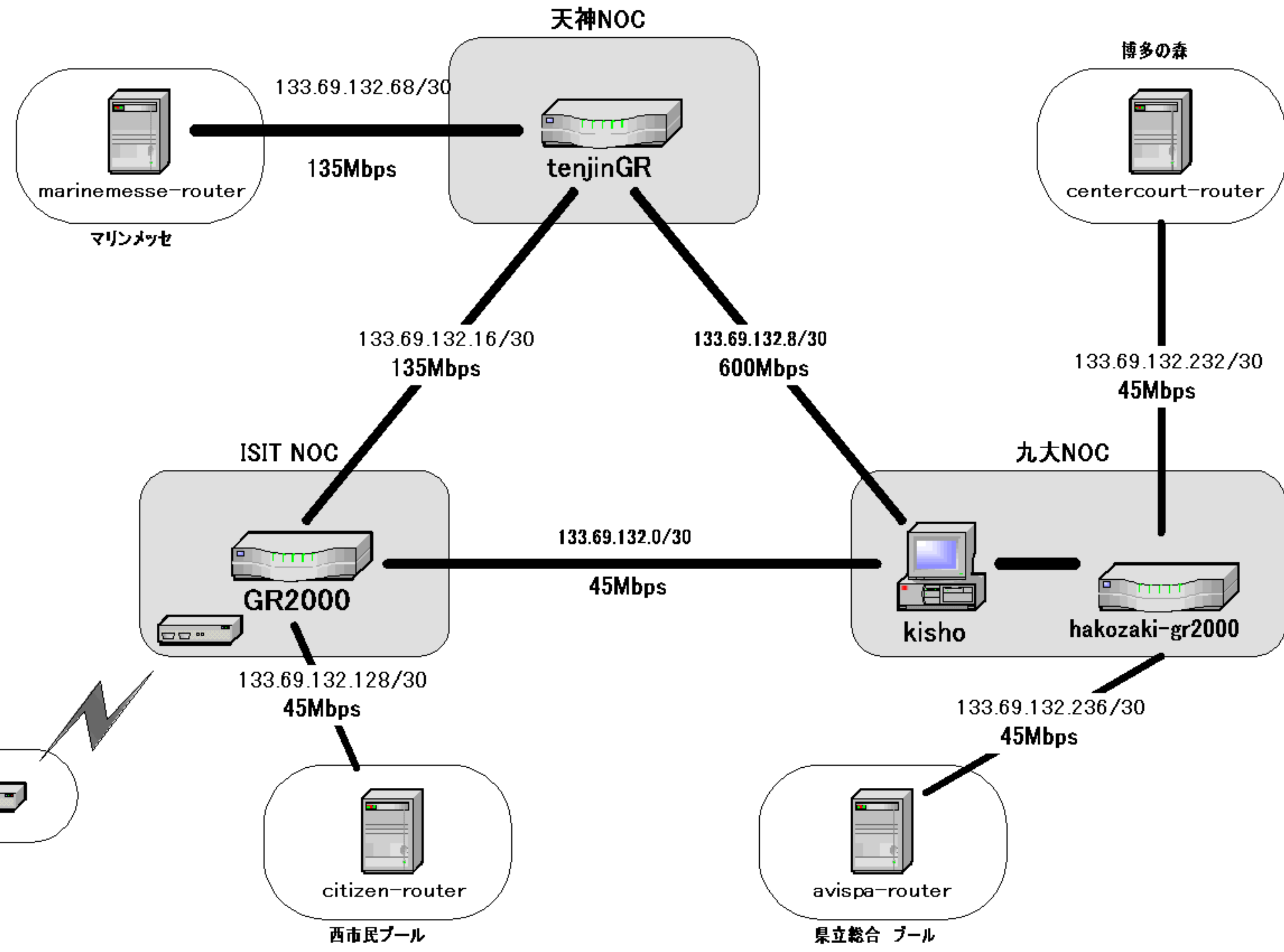
図1 ネットワーク構成
